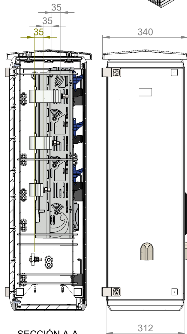
SECCIÓN A-A ESCALA 1 : 9
