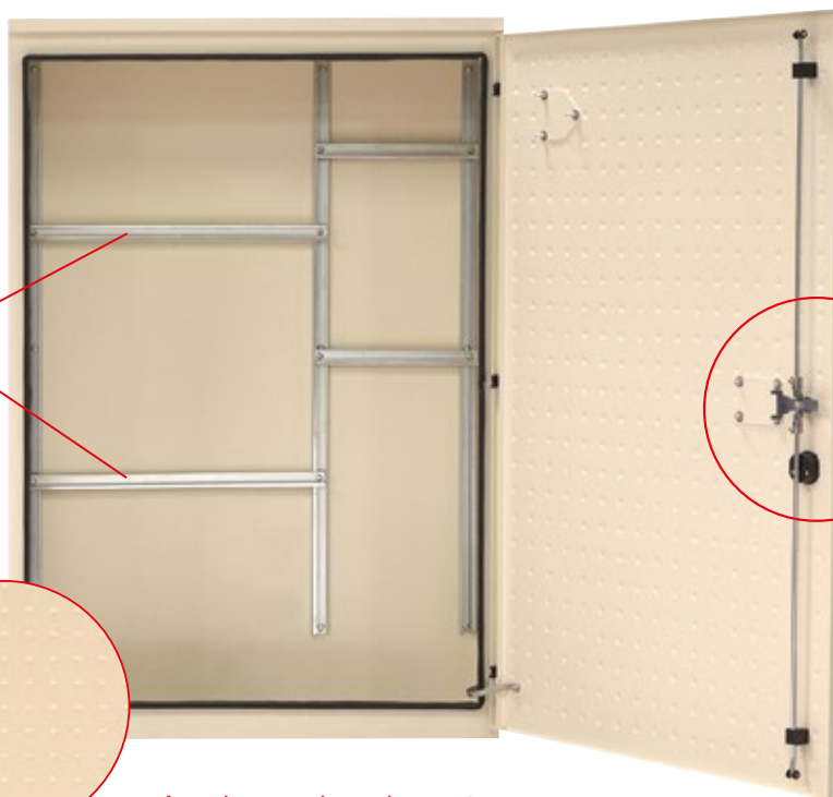
Armoire pour branchement à puissance surveillée Réf. 0460.505
