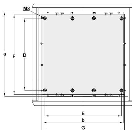
Plaque de montage (mm)
