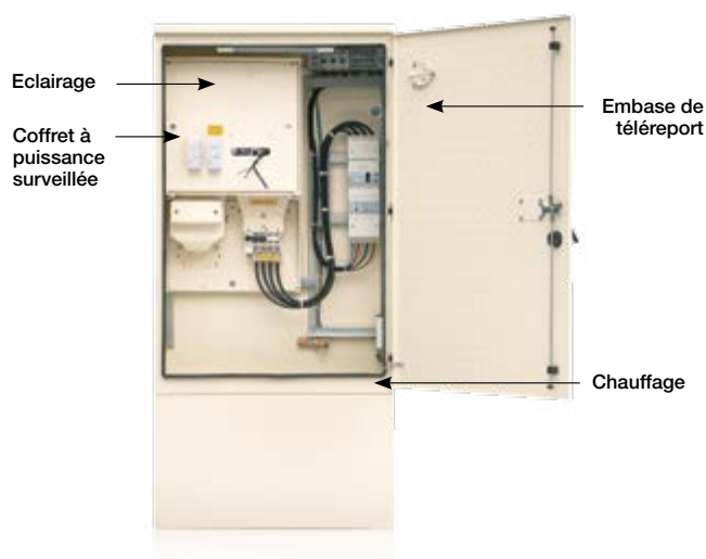
Armoire équipée pour branchement à puissance surveillée
