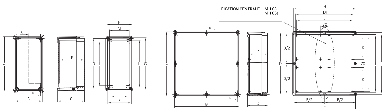
Dimensions Boîtiers (mm)
