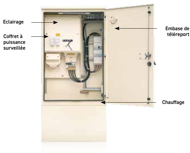
Armoire équipée pour branchement à puissance surveillée
