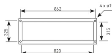
Schéma d'implantation au sol
