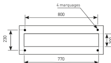
Schéma d'implantation au sol
