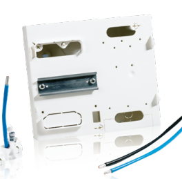
Panneau de comptage mono Type A
