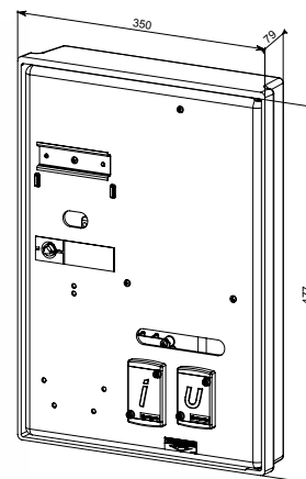
Coffret tableau PME-PMI
